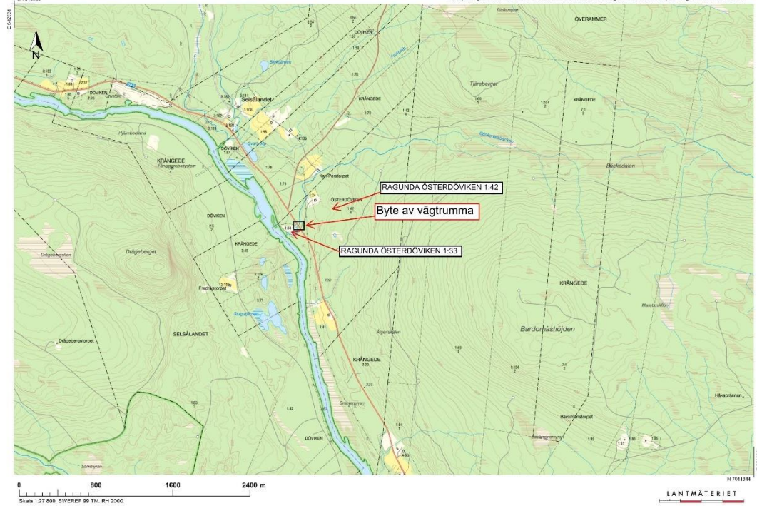
Figur 1, Plats för vägtrumma som skall bytas.
